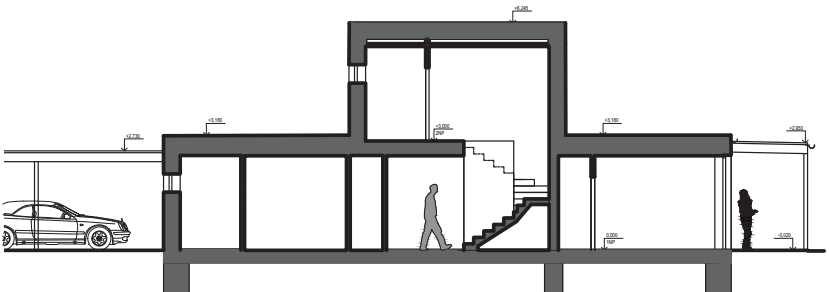
ŘEZA-A
