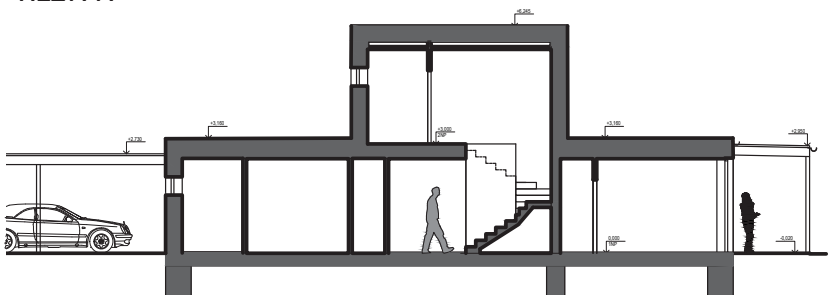
ŘEZ A-A
