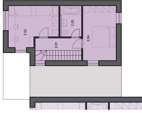
2.NP
